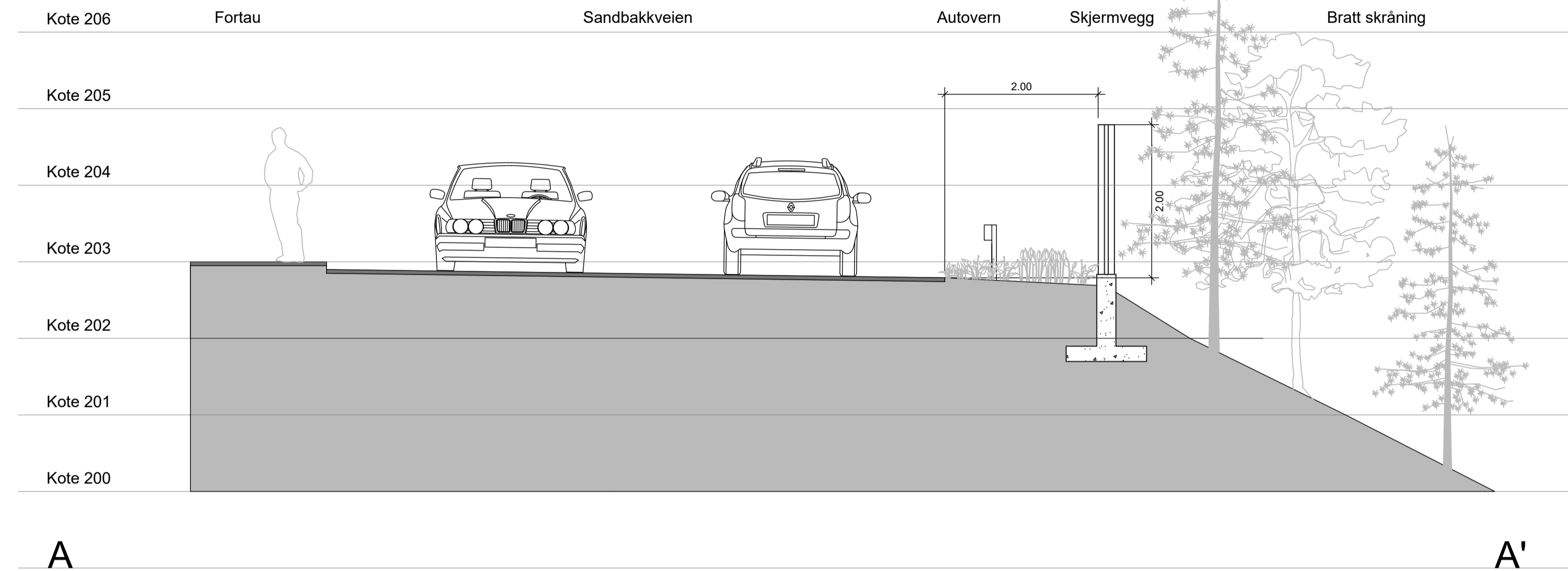
Snitt A-A' : Tverrsnitt veg, autovern og støyskjerm Målestokk - 1:50 i A1 1:100 i A3
